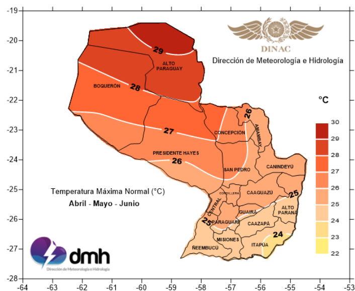
Figura 10. Temperatura máxima media normal. AMJ.
