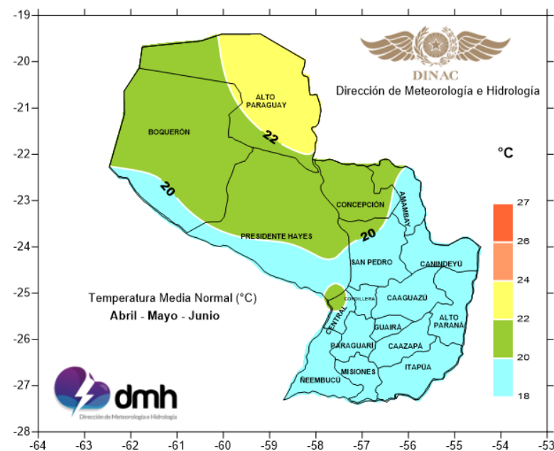
Figura 9. Temperatura media normal. AMJ.
