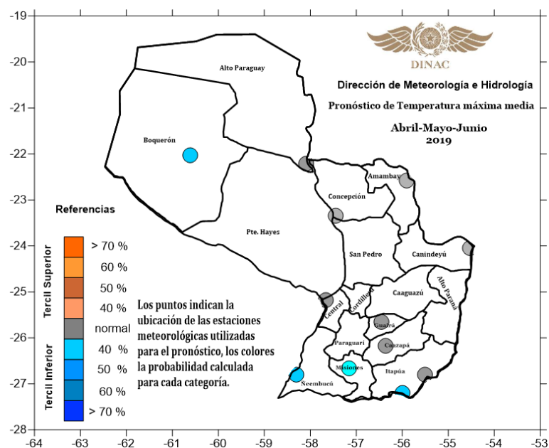
Figura 6. Pronóstico de temperatura máxima media. AMJ 2019.
