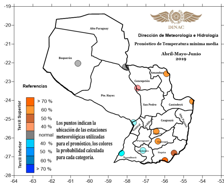
Figura 7. Pronóstico de temperatura mínima media. AMJ 2019.
