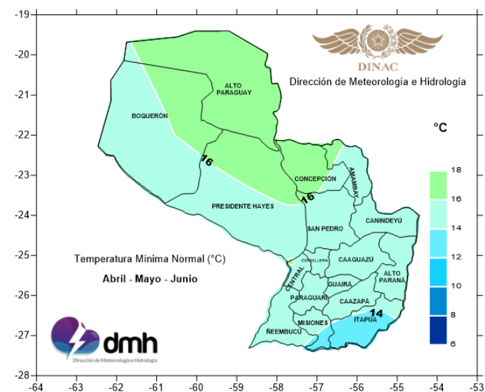
Figura 11. Temperatura mínima media normal. AMJ.
