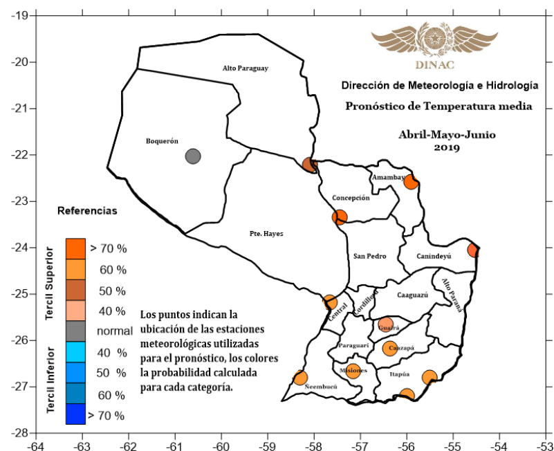
Figura 5. Pronóstico de Temperatura media trimestre AMJ 2019.
