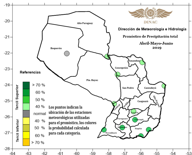
Figura 4. Pronóstico de Precipitación trimestre AMJ 2019.
