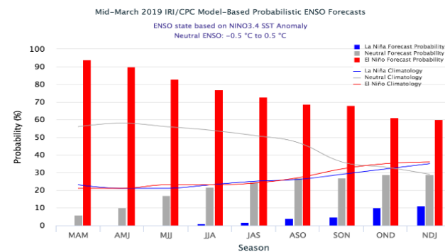
Figura 2. Probabilidad de fases del ENSO para la región de El Niño 3.4 actualizado al 19 de marzo de 2019. Fuente: IRI (Instituto Internacional de Investigación para el Clima y La Sociedad).
