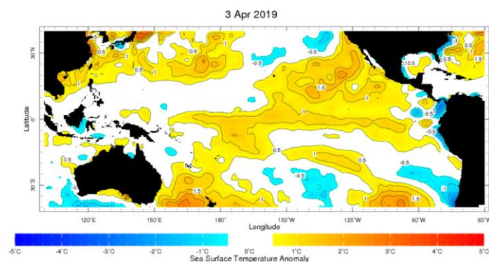
Figura 1. Anomalía de la temperatura superficial del mar en °C promediada en la semana del 31 de marzo al 03 de abril de 2019. Fuente: IRI. (Instituto Internacional de Investigación para el Clima y La Sociedad).
