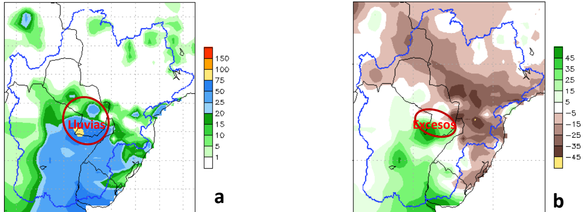
Figura 2: a) Cantidad de lluvia prevista (en mm) desde el 09 al 15 de junio. b) Anomalia de lluvia acumulada desde el 09 al 15 de junio. En él se pueden determinar las zonas con posibles excesos (verde) o déficits (marrón) de lluvias previstas para esas fechas. Fuente: NOAA.
