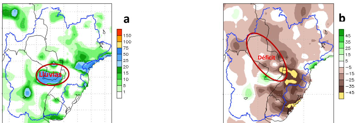
Figura 1: a) Cantidad de lluvia prevista (en mm) desde el 2 al 8 de junio. b) Anomalía de lluvia acumulada (en mm) desde el 2 al 8 de junio. En él se pueden determinar las zonas con posibles excesos (verde) o déficits (marrón) de lluvias previstas para esas fechas. Fuente: NOAA.
