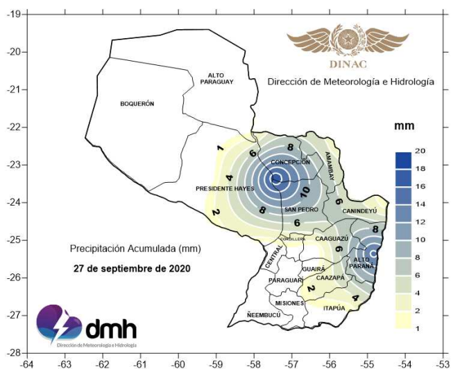
Figura 1. Precipitación total acumulada 27 de setiembre 2020
