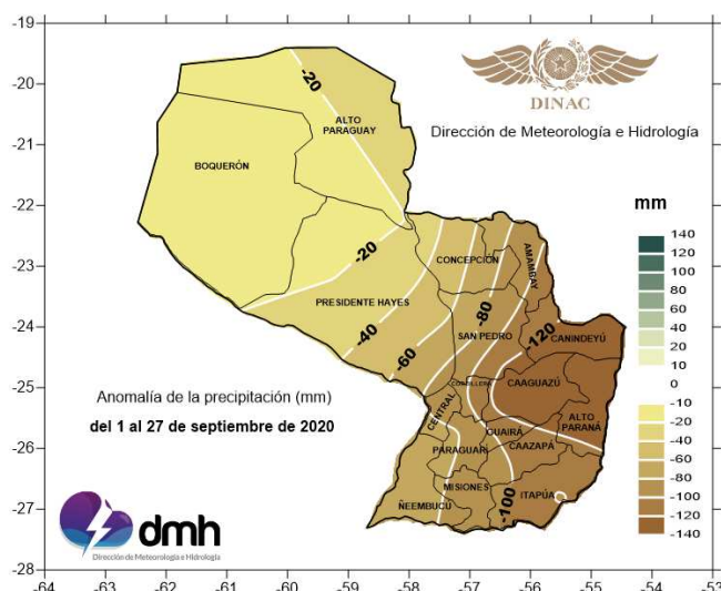
Figura 2. Anomalia de precipitación mensual de setiembre 2020
