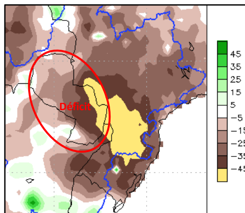
Figura 2: a) Cantidad de lluvia prevista (en mm) desde el 26 de abril al 02 de mayo. b) Anomalía de lluvia acumulada desde el 26 de abril al 02 de mayo. En él se pueden determinar las zonas con posibles excesos (verde) o déficits (marrón) de lluvias previstas para esas fechas. Fuente: NOAA.
