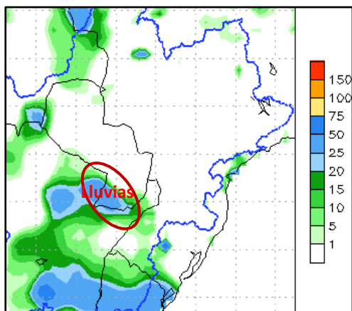
Figura 2: a) Cantidad de lluvia prevista (en mm) desde el 26 de abril al 02 de mayo. b) Anomalía de lluvia acumulada desde el 26 de abril al 02 de mayo. En él se pueden determinar las zonas con posibles excesos (verde) o déficits (marrón) de lluvias previstas para esas fechas. Fuente: NOAA.
