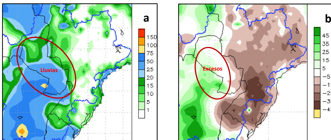
Figura 1: a) Cantidad de lluvia prevista (en mm) desde el 19 al 25 de abril b) Anomalia de lluvia acumulada (en mm) desde el 19 al 25 de abril. En él se pueden determinar las zonas con posibles excesos (verde) o déficits (marrón) de lluvias previstas para esas fechas. Fuente: NOAA.
