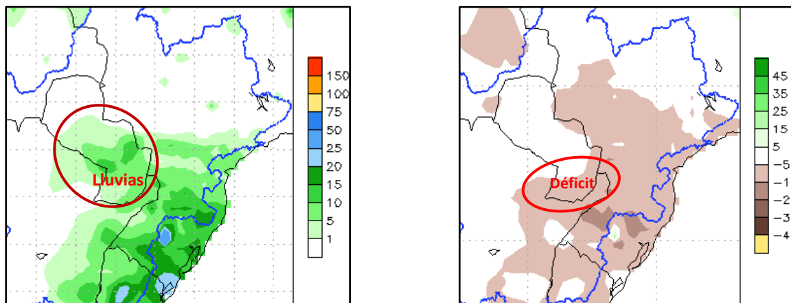
Figura 2: a) Cantidad de lluvia prevista (en mm) desde el 09 a 15 de agosto. b) Anomalia de lluvia acumulada desde el 09 a 15 de agosto. En él se pueden determinar las zonas con posibles excesos (verde) o déficits (marrón) de lluvias previstas para esas fechas. Fuente: NOAA.
