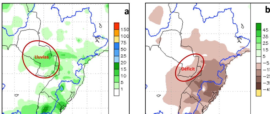
Figura 1: a) Cantidad de lluvia prevista (en mm) desde el 02 al 08 de agosto b) Anomalía de lluvia acumulada (en mm) desde el 02 al 08 de agosto. En él se pueden determinar las zonas con posibles excesos (verde) o déficits (marrón) de lluvias previstas para esas fechas. Fuente: NOAA.
