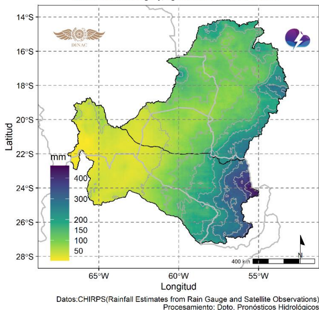
Figura 5. Precipitación total acumulada en milímetros.
