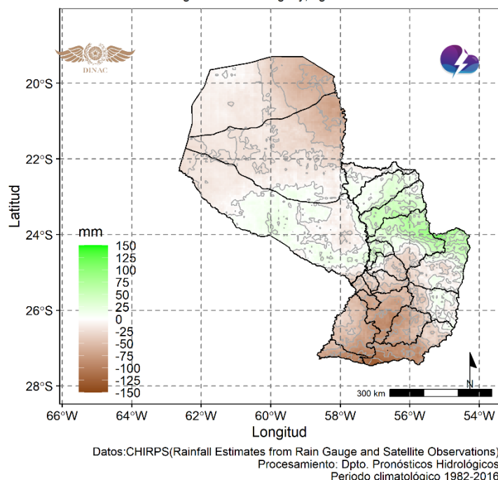
Figura 15. Anomalía de la precipitación en milímetros.
