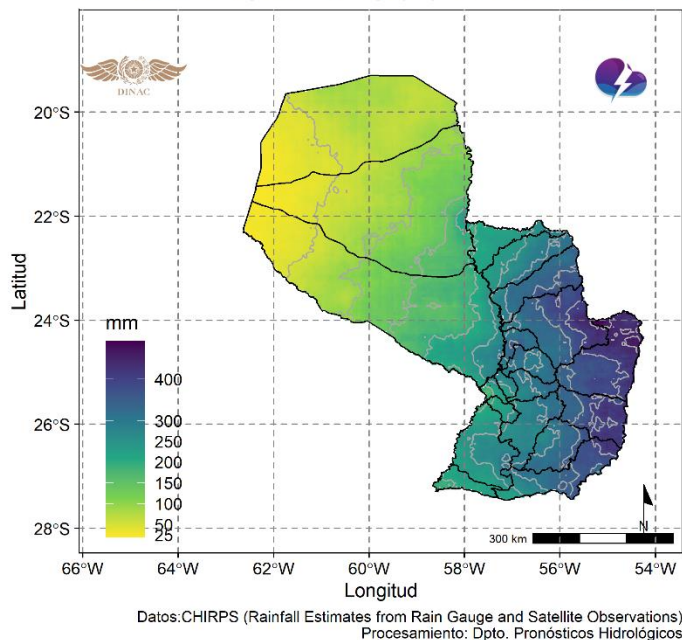
Figura 14. Precipitación total acumulada en milímetros.
