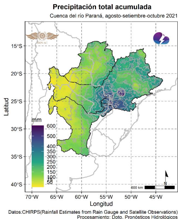
Figura 8. Precipitación total acumulada en milímetros.
