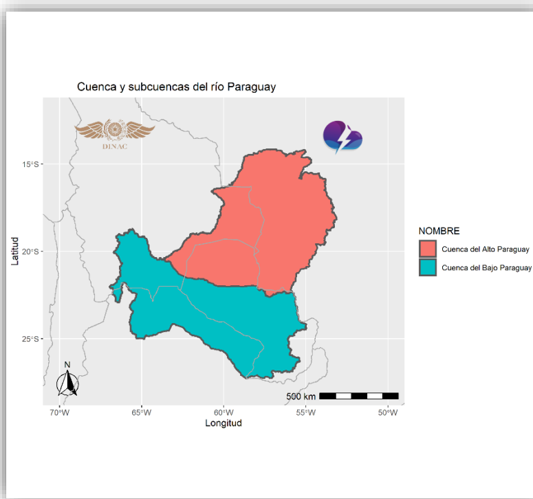
Figura 4. Cuenca y subcuencas del río Paraguay. Fuente: Departamento de pronósticos hidrológicos.
