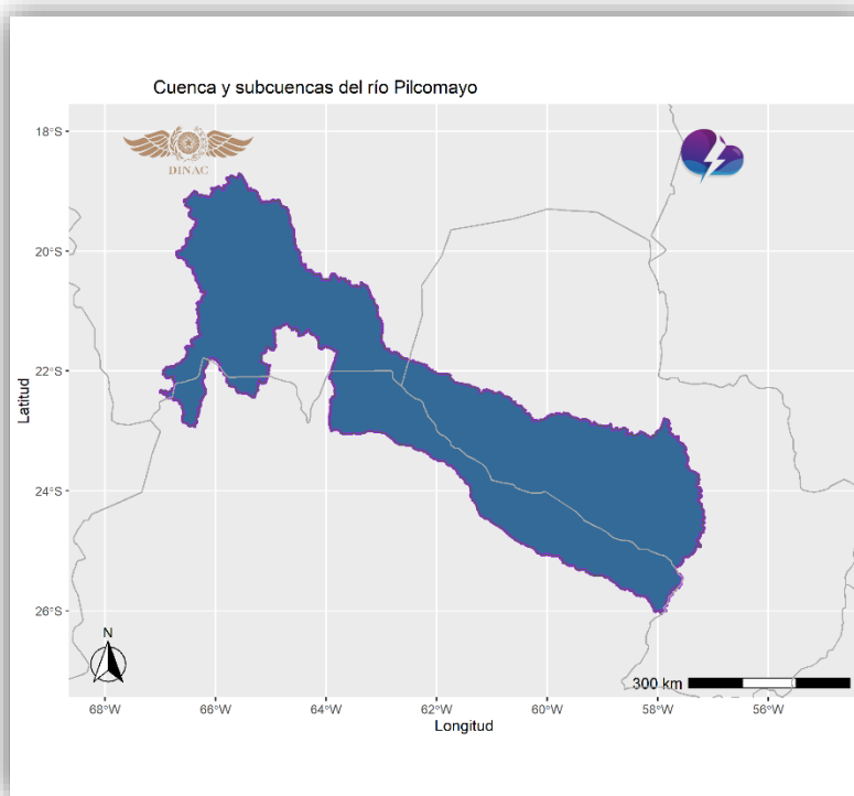
Figura 10. Cuenca y subcuencas del río Pilcomayo. Fuente: Departamento de pronósticos hidrológicos.
