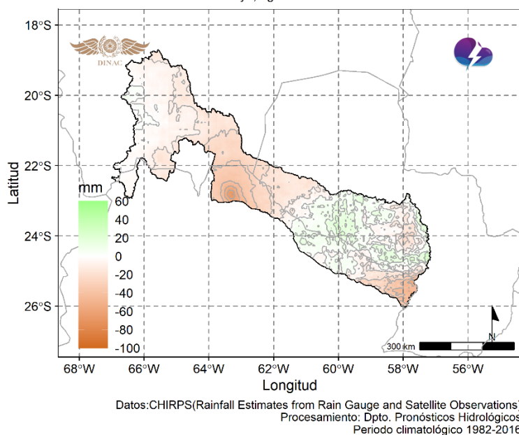
Figura 12. Anomalía de la precipitación en milímetros.
