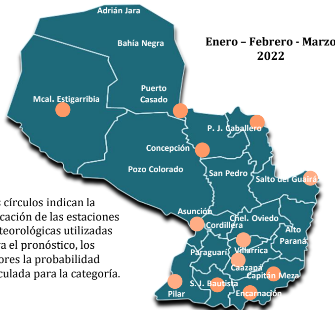
Figura 6. Pronóstico de temperatura máxima media. EFM 2022.
