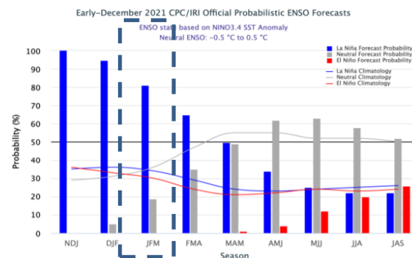
Figura 2. Probabilidad de fases del ENSO para la región de El Niño 3.4 actualizado al 9 de diciembre de 2021. Fuente: IRI (Instituto Internacional de Investigación para el Clima y La Sociedad).
