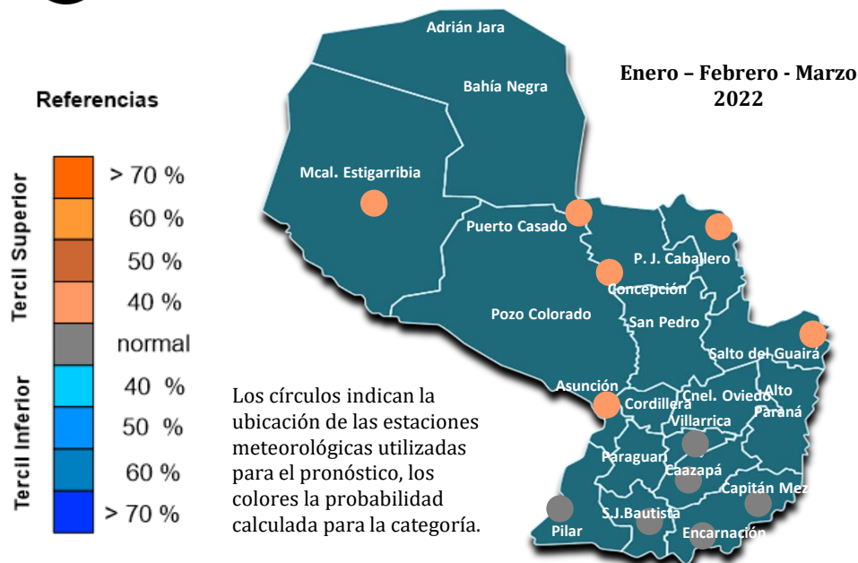
Figura 7. Pronóstico de temperatura mínima media. EFM 2022.
