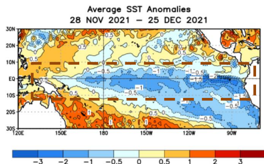
Figura 1. Anomalía de la temperatura superficial del mar en °C promediada en la semana del 28 de noviembre al 25 de diciembre de 2021. Fuente: IRI. (Instituto Internacional de Investigación para el Clima y la Sociedad).
