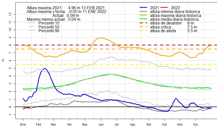
Altura diaria del río Paraguay, Villeta
