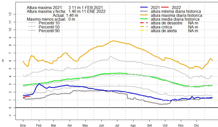
Altura diaria del río Paraguay, Vallemi
