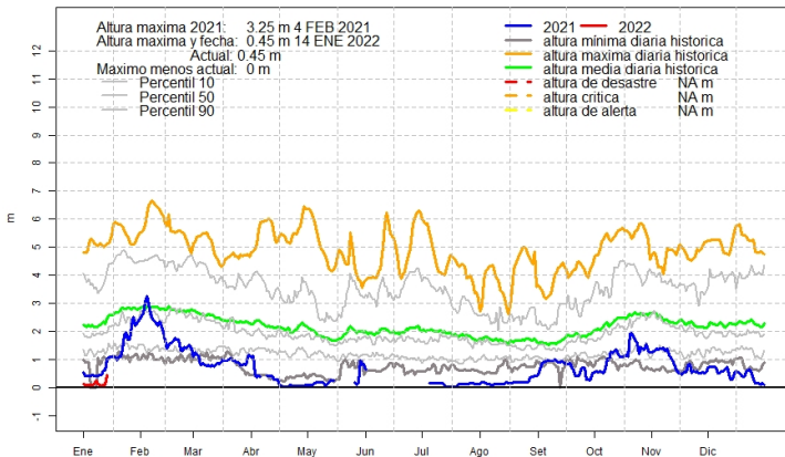
Altura diaria del río Paraná, Ayolas
