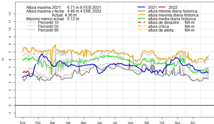
Altura diaria del río Paraná, Salto del Guaira
