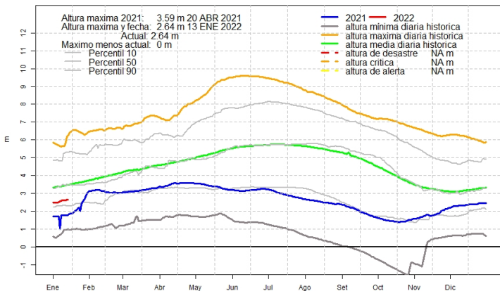
Altura diaria del río Paraguay, Fuerte Olimpo
