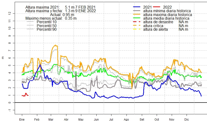
Altura diaria del río Paraná, Ita Piru
