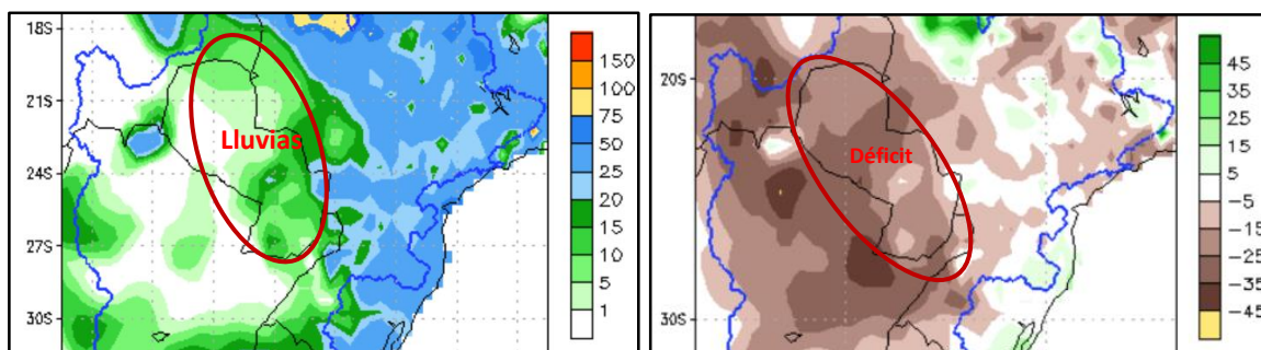
Figura 2: a) Cantidad de lluvia prevista (en mm) desde el 13 al 19 de marzo b) Anomalía de lluvia acumulada desde el 13 al 19 de marzo. En él se pueden determinar las zonas con posibles excesos (verde) o déficits (marrón) de lluvias previstas para esas fechas. Fuente: NOAA.
