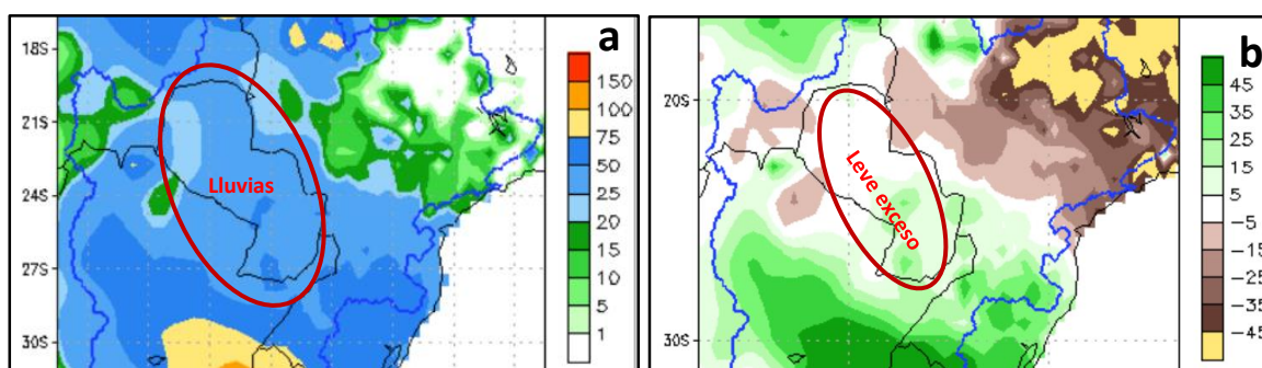
Figura 1: a) Cantidad de lluvia prevista (en mm) desde el 06 al 12 de marzo b) Anomalía de lluvia acumulada (en mm) desde el 06 al 12 de marzo. En él se pueden determinar las zonas con posibles excesos (verde) o déficits (marrón) de lluvias previstas para esas fechas. Fuente: NOAA.
