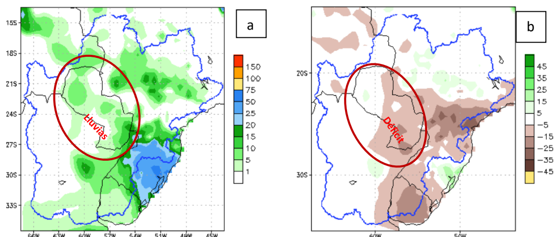
Figura 1: a) Cantidad de lluvia prevista (en mm) desde el 02 al 08 de julio. b) Anomalía de lluvia acumulada (en mm) desde el 02 al 08 de julio. En él se pueden determinar las zonas con posibles excesos (verde) o déficits (marrón) de lluvias previstas para esas fechas. Fuente: NOAA.
