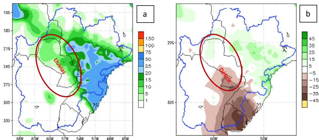
Figura 2: a) Cantidad de lluvia prevista (en mm) desde el 09 al 15 de julio. b) Anomalía de lluvia acumulada desde el 09 al 15 de julio. En él se pueden determinar las zonas con posibles excesos (verde) o déficits (marrón) de lluvias previstas para esas fechas. Fuente: NOAA.
