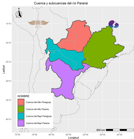
Figura 7: Cuenca del río Paraná.
