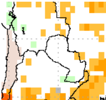
Anomalía de la precipitación, trimestre: agosto-setiembre-octubre, modelo NMME-NOAA
