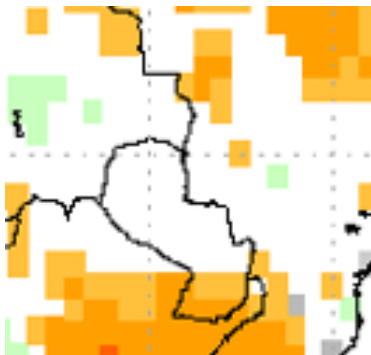
Anomalía de la precipitación, trimestre: Octubre-Noviembre-Diciembre, modelo NMME-NOAA
