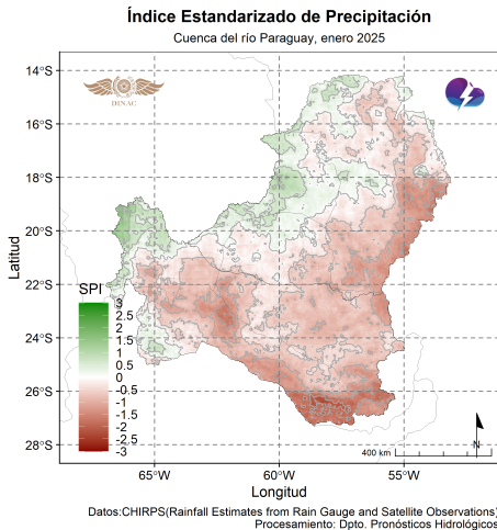
Figura 24: Índice Estandarizado de Precipitación mensual. Fuente: DPH-DMH.
