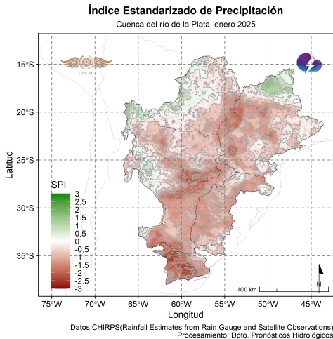
Figura 23: Índice Estandarizado de Precipitación mensual. Fuente: DPH-DMH.
