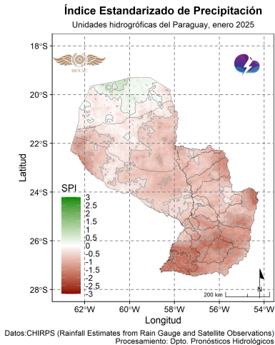
Figura 27: Índice Estandarizado de Precipitación mensual. Fuente: DPH-DMH.
