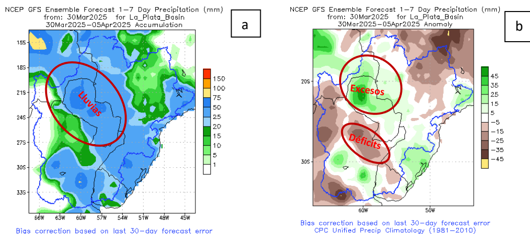
Figura 1: a) Cantidad de lluvia prevista (en mm) desde el 30 de marzo al 05 de abril . b) Anomalía de lluvia acumulada (en mm) desde el 30 de marzo al 05 de abril . En él se pueden determinar las zonas con posibles excesos (verde) o déficits (marrón) de lluvias previstas para esas fechas. Fuente: NOAA.
