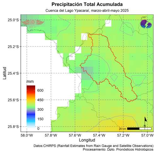
Figura 17: Precipitación total trimestral. Fuente: DPH-DMH.
