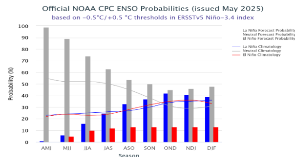
Figura 2. Probabilidad de fases del ENSO para la región de El Niño 3.4 actualizado al 19 de mayo de 2025. Fuente: IRI (Instituto Internacional de Investigación para el Clima y La Sociedad).
