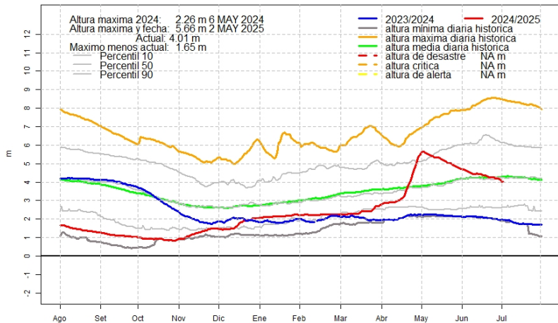
Altura diaria del río Paraguay, Vallemit
