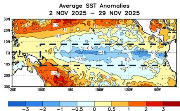
Figura 1. Anomalía de la temperatura superficial del mar en °C promediada en la semana del 02 de noviembre al 29 de noviembre de 2025. Fuente: IRI. (Instituto Internacional de Investigación para el Clima y la Sociedad).
