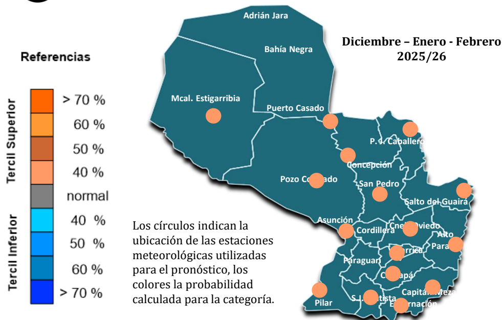
Figura 7. Pronóstico de temperatura mínima media. DEF 2025/26.
