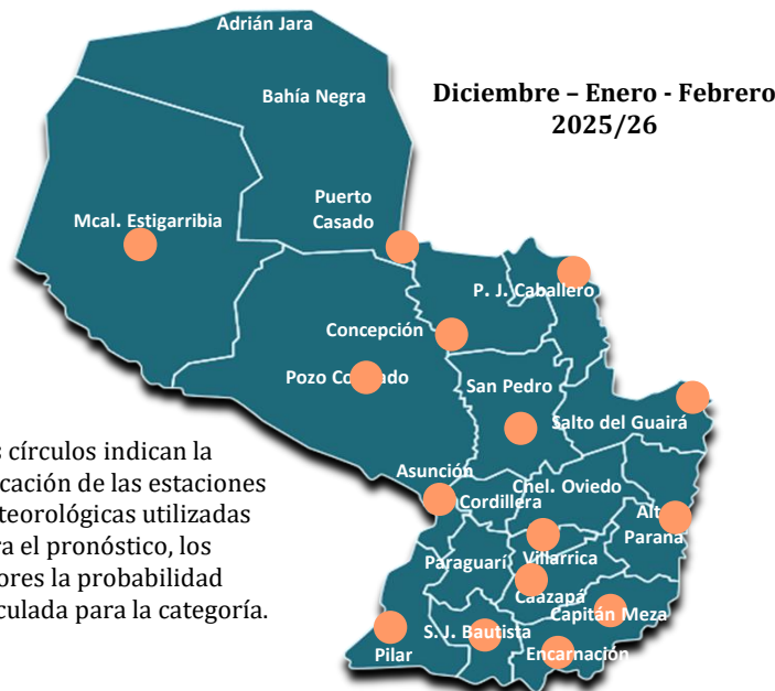
Figura 6. Pronóstico de temperatura máxima media. DEF 2025/26.
