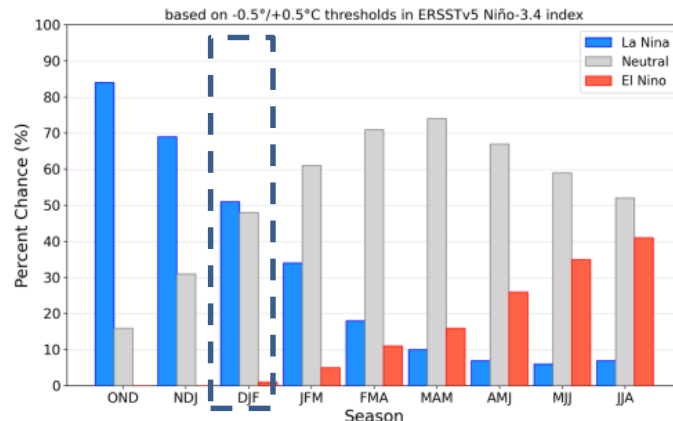
Figura 2. Probabilidad de fases del ENSO para la región de El Niño 3.4 actualizado al 13 de noviembre de 2025. Fuente: IRI (Instituto Internacional de Investigación para el Clima y La Sociedad).
