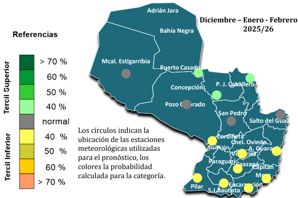
Figura 4. Pronóstico de Precipitación trimestre DEF 2025/26.
