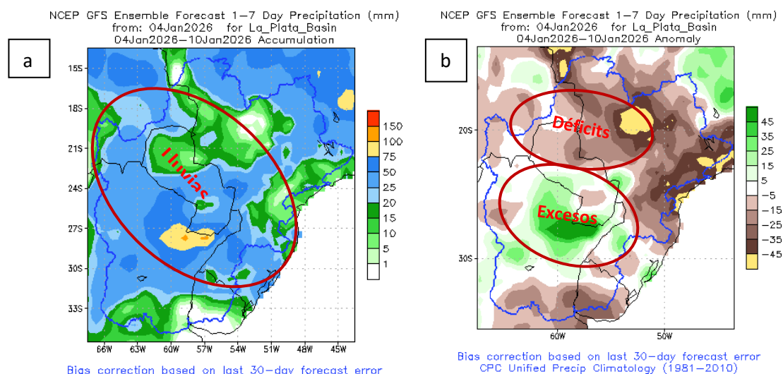
Figura 1: a) Cantidad de lluvia prevista (en mm) desde el 04 al 10 de enero . b) Anomalía de lluvia acumulada (en mm) desde el 04 al 10 de enero . En él se pueden determinar las zonas con posibles excesos (verde) o déficits (marrón) de lluvias previstas para esas fechas. Fuente: NOAA.
