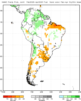
Anomalía, trimestre Feb-Mar-Abr, modelo NMME-NOAA
