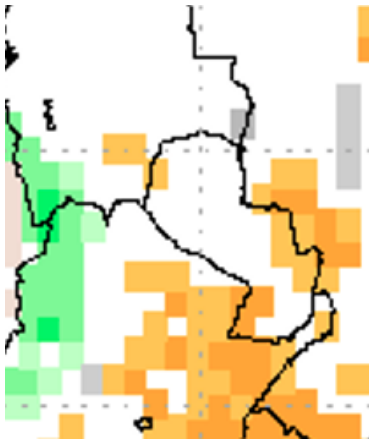
Anomalía, trimestre Feb-Mar-Abr, modelo NMME-NOAA
