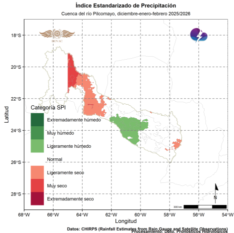
Figura 26: Índice Estandarizado de Precipitación trimestral. Fuente: DPH-DMH.
