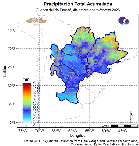
Figura 8: Precipitación total trimestral. Fuente: DPH-DMH.
