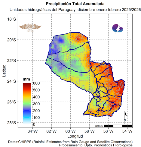
Figura 14: Precipitación total trimestral. Fuente: DPH-DMH.
