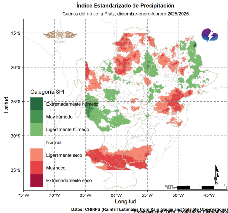
Figura 23: Índice Estandarizado de Precipitación trimestral. Fuente: DPH-DMH.
