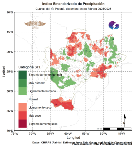
Figura 25: Índice Estandarizado de Precipitación trimestral. Fuente: DPH-DMH.
