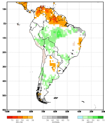
Anomalía, trimestre May-Jun-Jul, modelo NMME-NOAA
