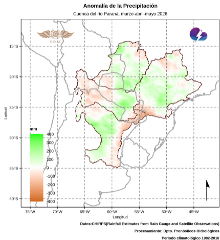
Figura 9: Anomalia de la precipitación trimestral. Fuente: DPH-DMH.
