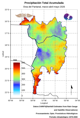
Figura 20: Precipitación total mensual. Fuente: DPH-DMH.
