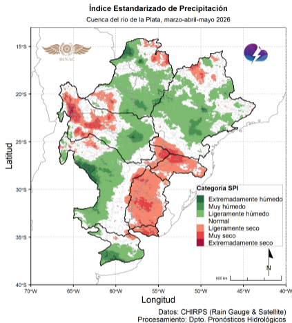
Figura 23: Índice Estandarizado de Precipitación trimestral. Fuente: DPH-DMH.
