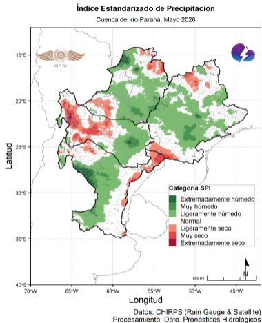
Figura 25: Índice Estandarizado de Precipitación trimestral. Fuente: DPH-DMH.
