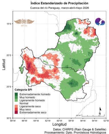
Figura 24: Índice Estandarizado de Precipitación trimestral. Fuente: DPH-DMH.
