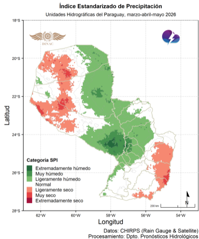
Figura 27: Índice Estandarizado de Precipitación trimestral. Fuente: DPH-DMH.
