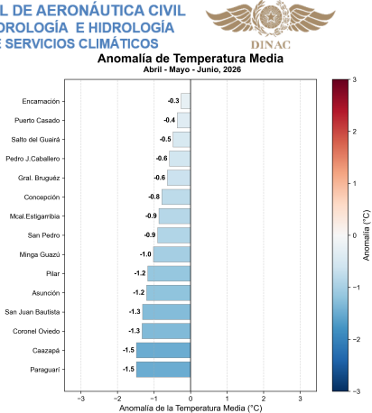
Figura 6. Anomalía de la temperatura media trimestral
