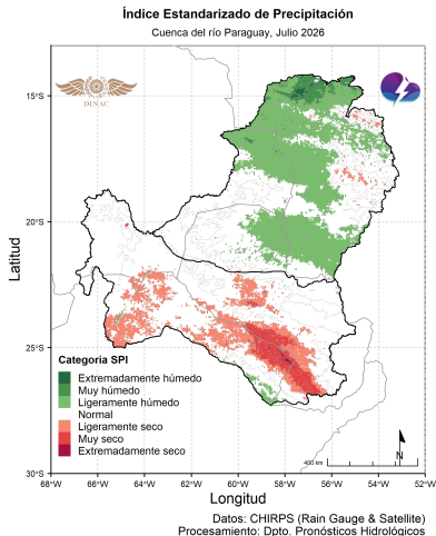
Figura 24: Índice Estandarizado de Precipitación mensual. Fuente: DPH-DMH.
