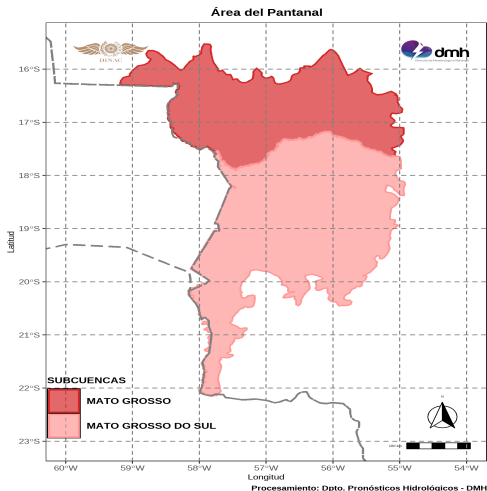
Figura 19: Cuenca del Pantanal. Fuente: DPH-DMH.
