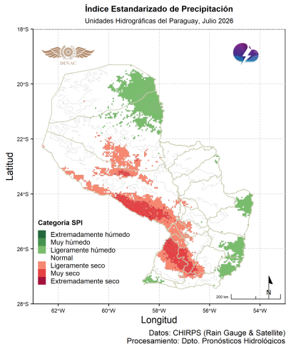
Figura 27: Índice Estandarizado de Precipitación mensual. Fuente: DPH-DMH.
