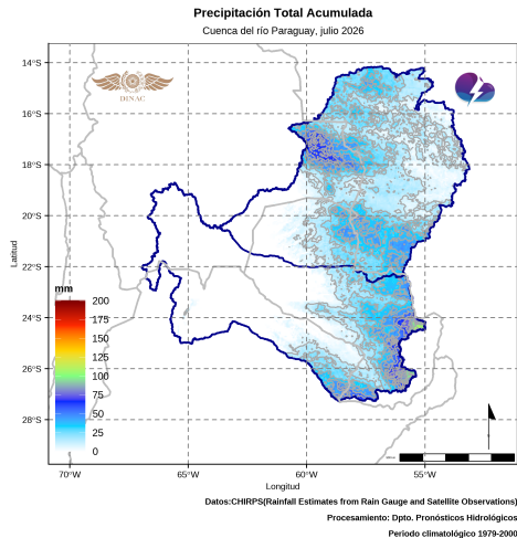
Figura 5: Precipitación total mensual. Fuente: DPH-DMH.
