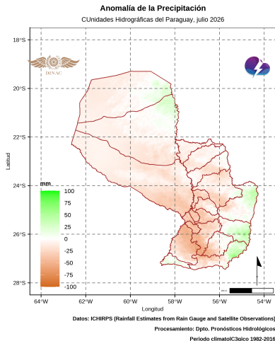
Figura 15: Anomalía de la precipitación mensual. Fuente: DPH-DMH.
