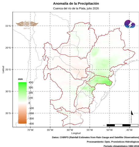
Figura 3: Anomalía de la precipitación mensual. Fuente: DPH-DMH.
