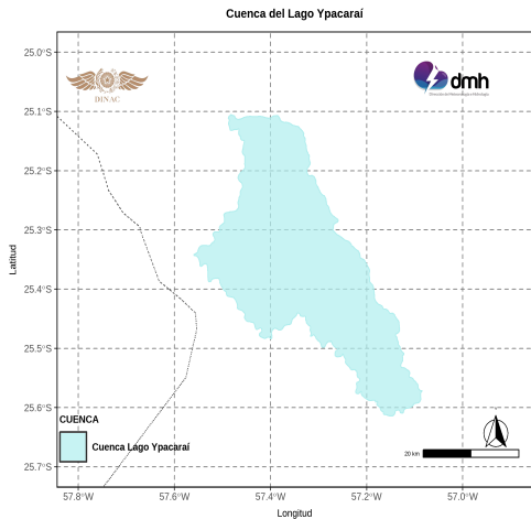
Figura 16: Cuenca del Lago Ypacaraí. Fuente: DPH-DMH.
