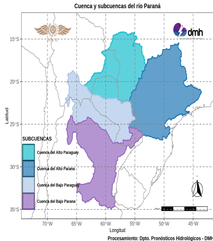
Figura 7: Cuenca del río Paraná. Fuente: DPH-DMH.
