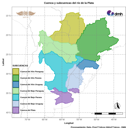
Figura 1: Cuenca del río de la Plata. Fuente: DPH-DMH.
