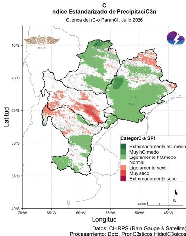
Figura 25: Índice Estandarizado de Precipitación mensual. Fuente: DPH-DMH.
