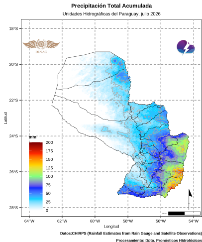
Figura 14: Precipitación total mensual. Fuente: DPH-DMH.
