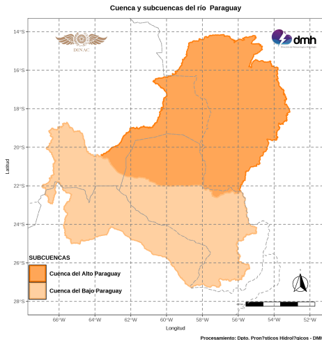
Figura 4: Cuenca del río de Paraguay. Fuente: DPH-DMH.
