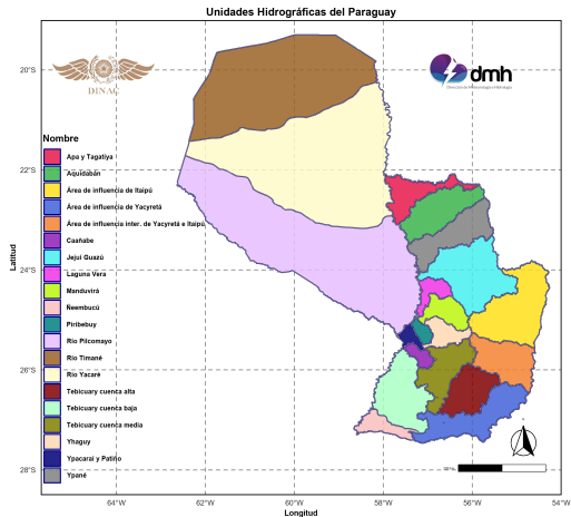
Figura 13: Unidades Hidrográficas del Paraguay. Fuente: DPH-DMH.
