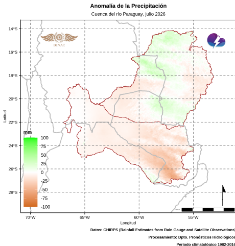
Figura 6: Anomalía de la precipitación mensual. Fuente: DPH-DMH.
