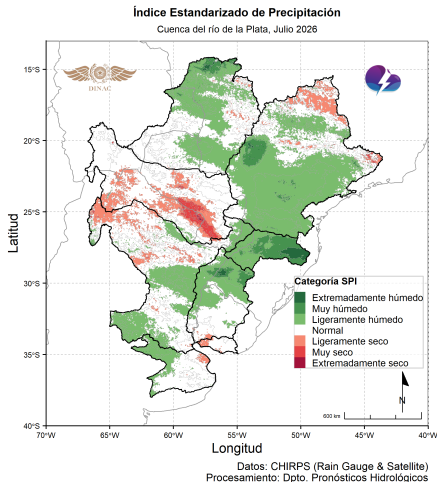
Figura 23: Índice Estandarizado de Precipitación mensual. Fuente: DPH-DMH.
