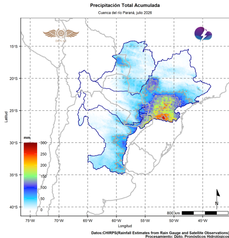
Figura 8: Precipitación total mensual. Fuente: DPH-DMH.
