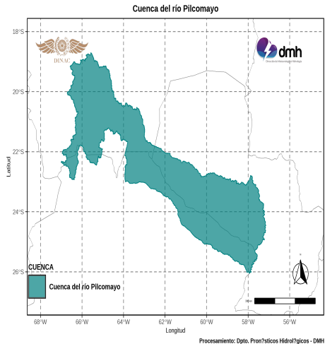
Figura 10: Cuenca del río Pilcomayo. Fuente: DPH-DMH.
