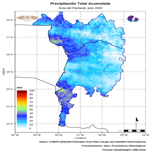
Figura 20: Precipitación total mensual. Fuente: DPH-DMH.
