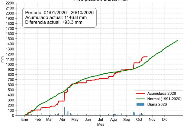
Precipitación diaria, Pilar
