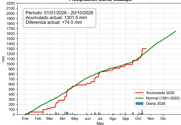
Precipitación diaria, Caazapa
