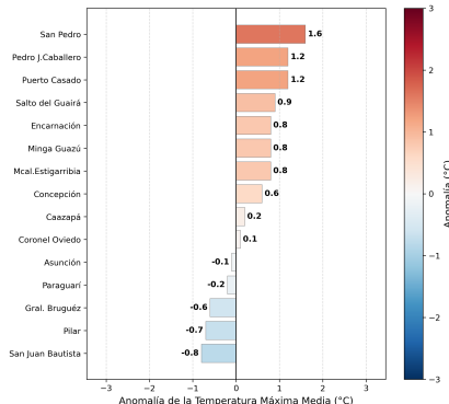
Figura 12. Anomalía de la temperatura máxima media trimestral
