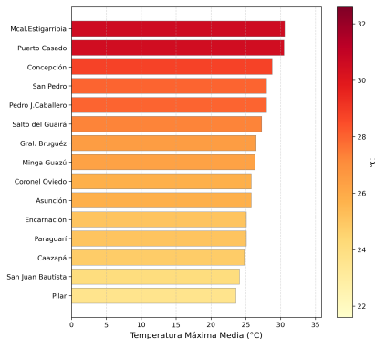
Figura 11. Temperatura máxima media trimestral
