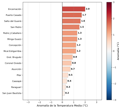
Figura 6. Anomalia de la temperatura media trimestral
